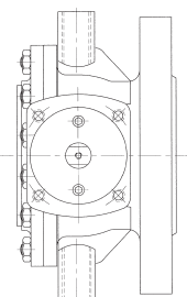
Tank bottom valve Fondo de cuba
