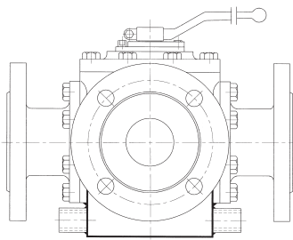
Three way valve Válvula de tres vías
